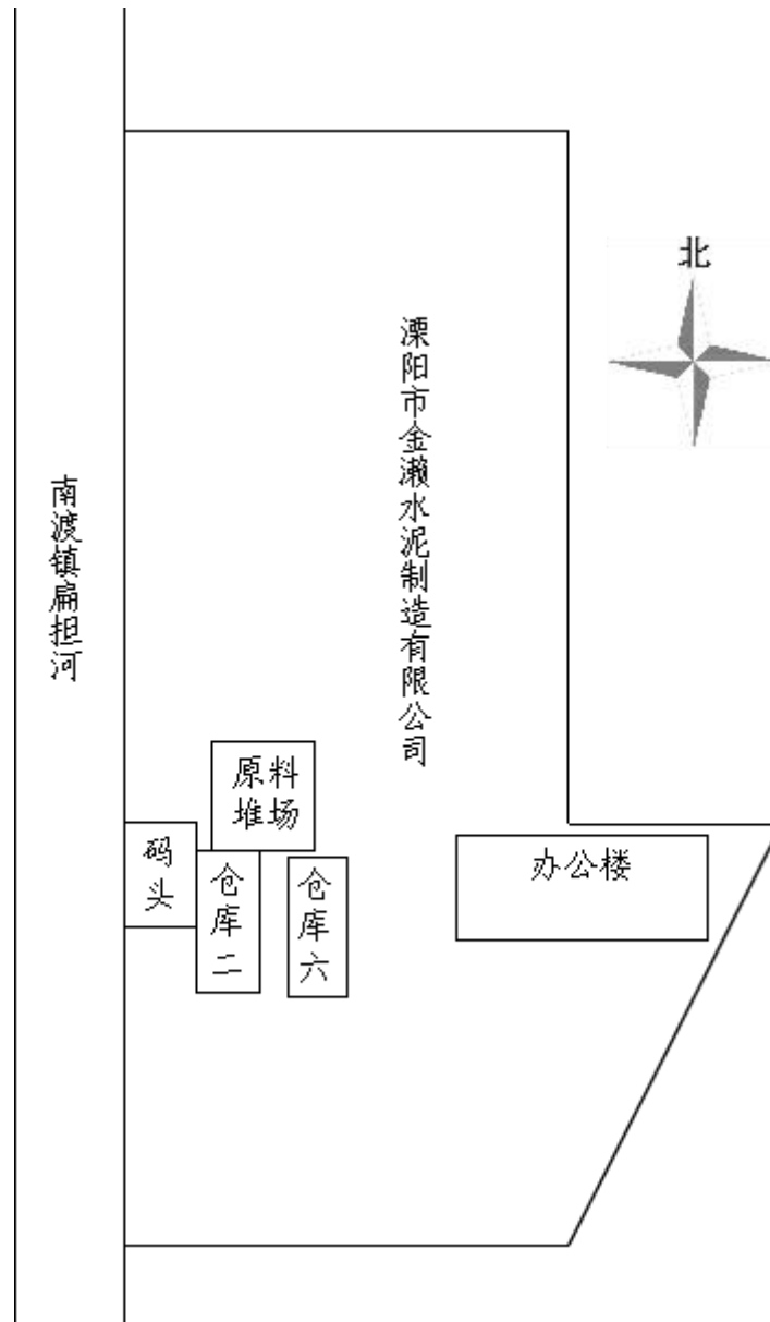
图4-3 厂区平面布置图
