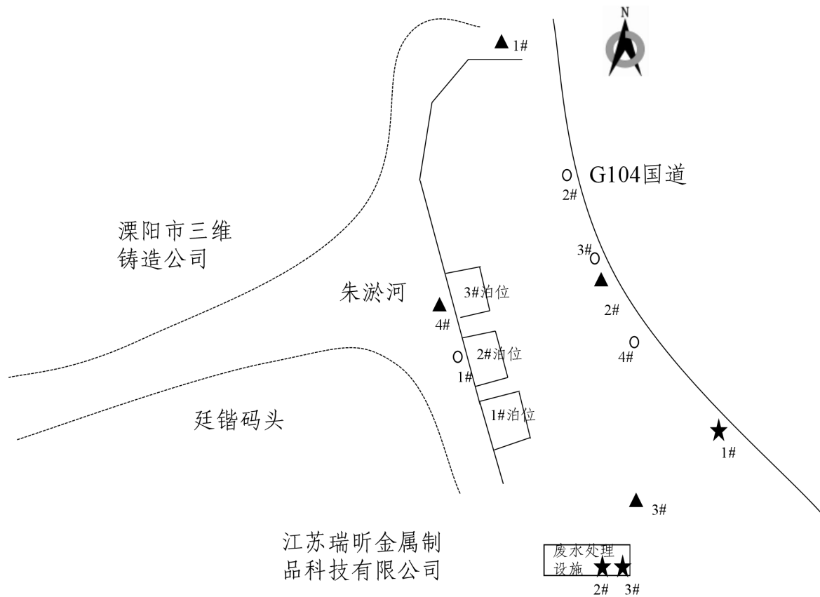
图 8-1 验收监测布点图示
