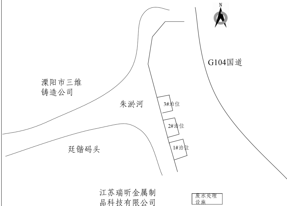
图4-3 厂区平面布置图
