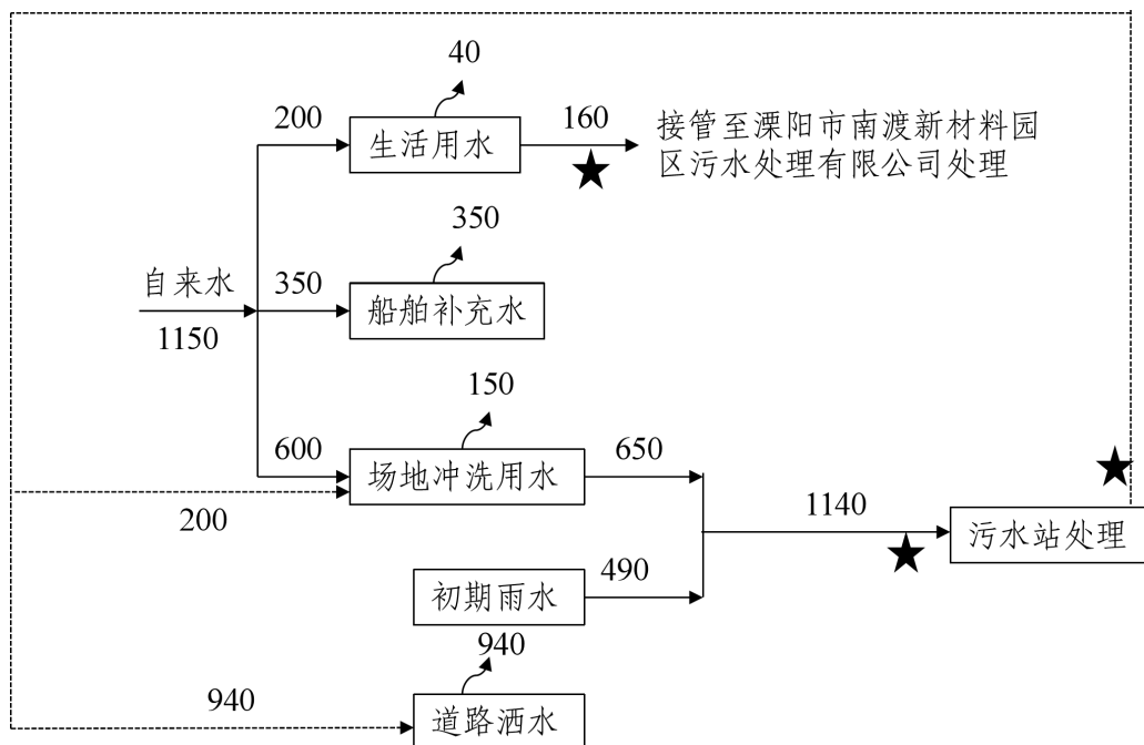
图 4-1 本项目水量及水平衡图 (t/a)
