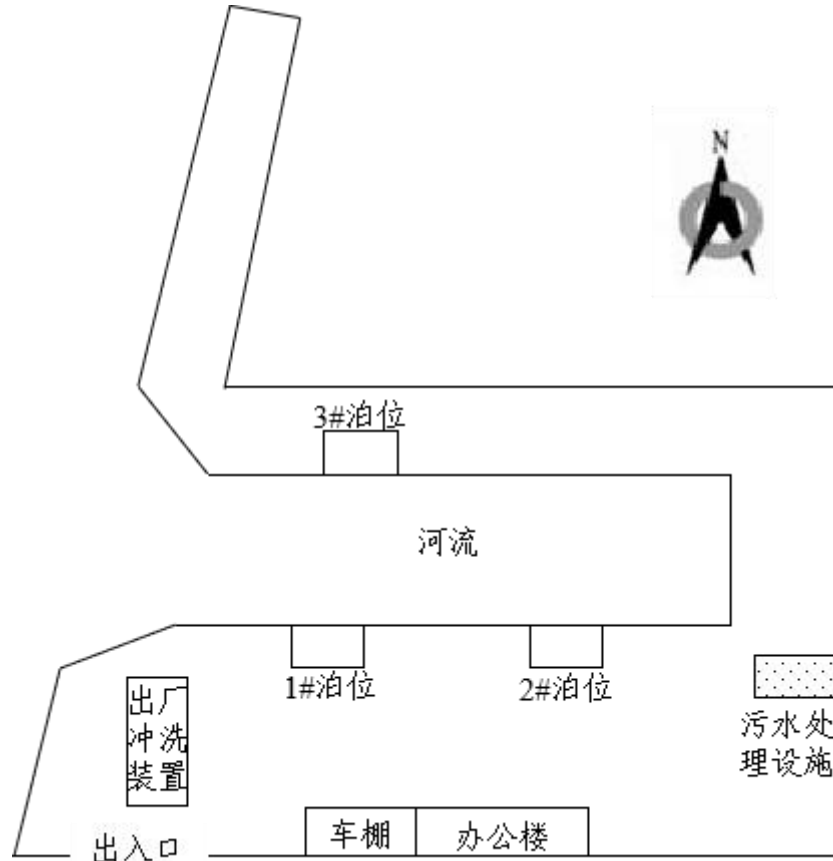
图4-3 厂区平面布置图
