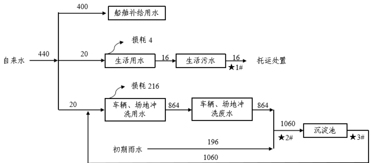
图 4-1 本项目水量及水平衡图 (t/a)
